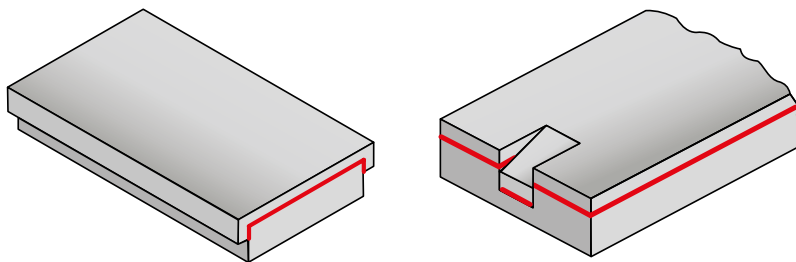
Abb. 39: Formschlüssige Befestigung von DP4-Gleitstreifen
