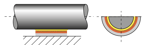
Abb. 24: Hydrodynamische Schmierung
