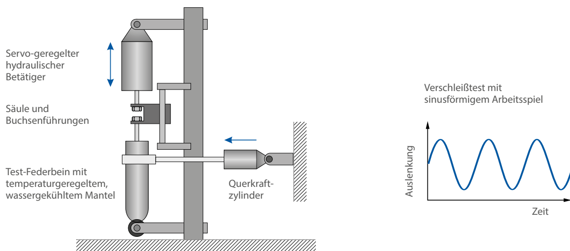
Abb. 7: Prinzipskizze des Testaufbaus
