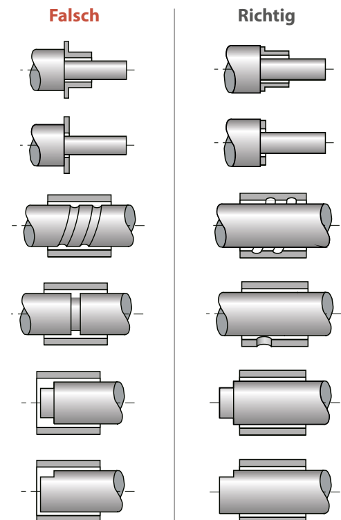
Abb. 31: Gestaltung der Gegenfläche
