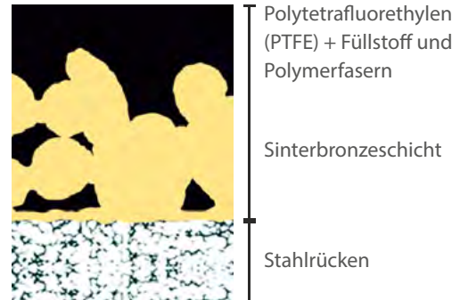
Abb.1: DP4 Mikroschliffbild
