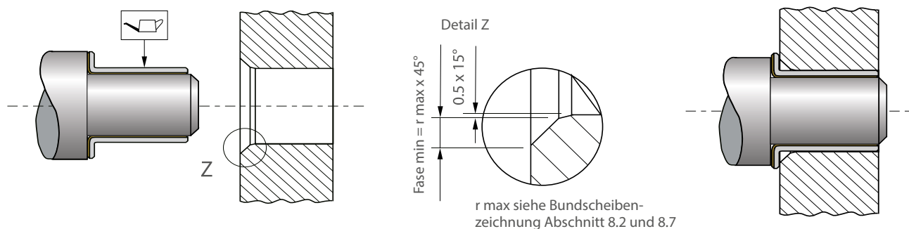
Abb. 33: Einpressen von Bundbuchsen
