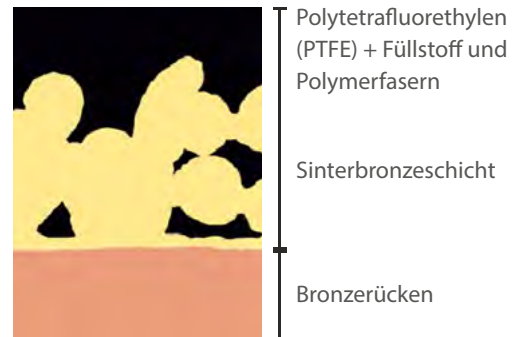
Abb. 2: DP4-B Mikroschliffbild
